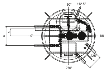
Exemple : Puits spécial avec deux pompes
