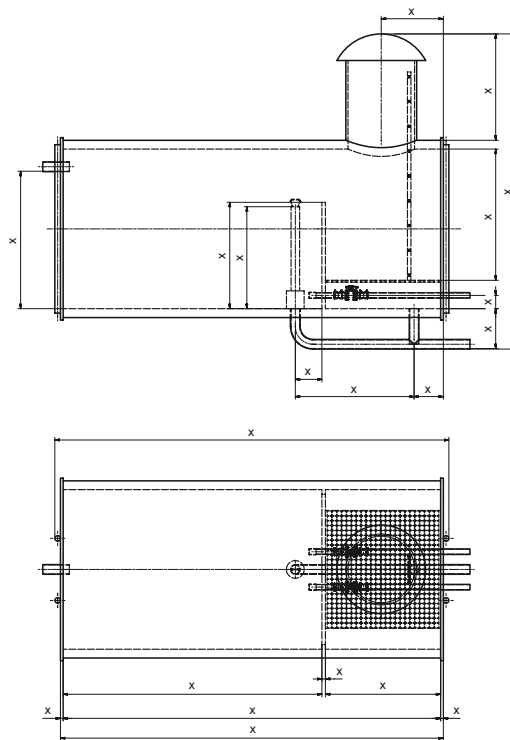
Exemple : Regard de rinçage
