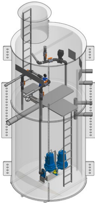
Beispiel: Grosser Pumpschacht mit Reservoirdeckel
