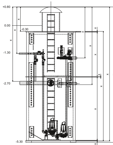
Exemple : Grand puits de pompe avec couvercle de réservoir
