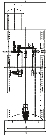
Esempio: Grande condotto per pompe con coperchio serbatoio
