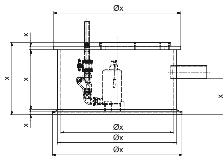
Exemple : Puits spécial avec deux pompes
